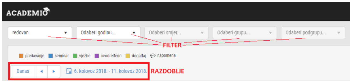
Slika 1. Filtriranje rasporeda
